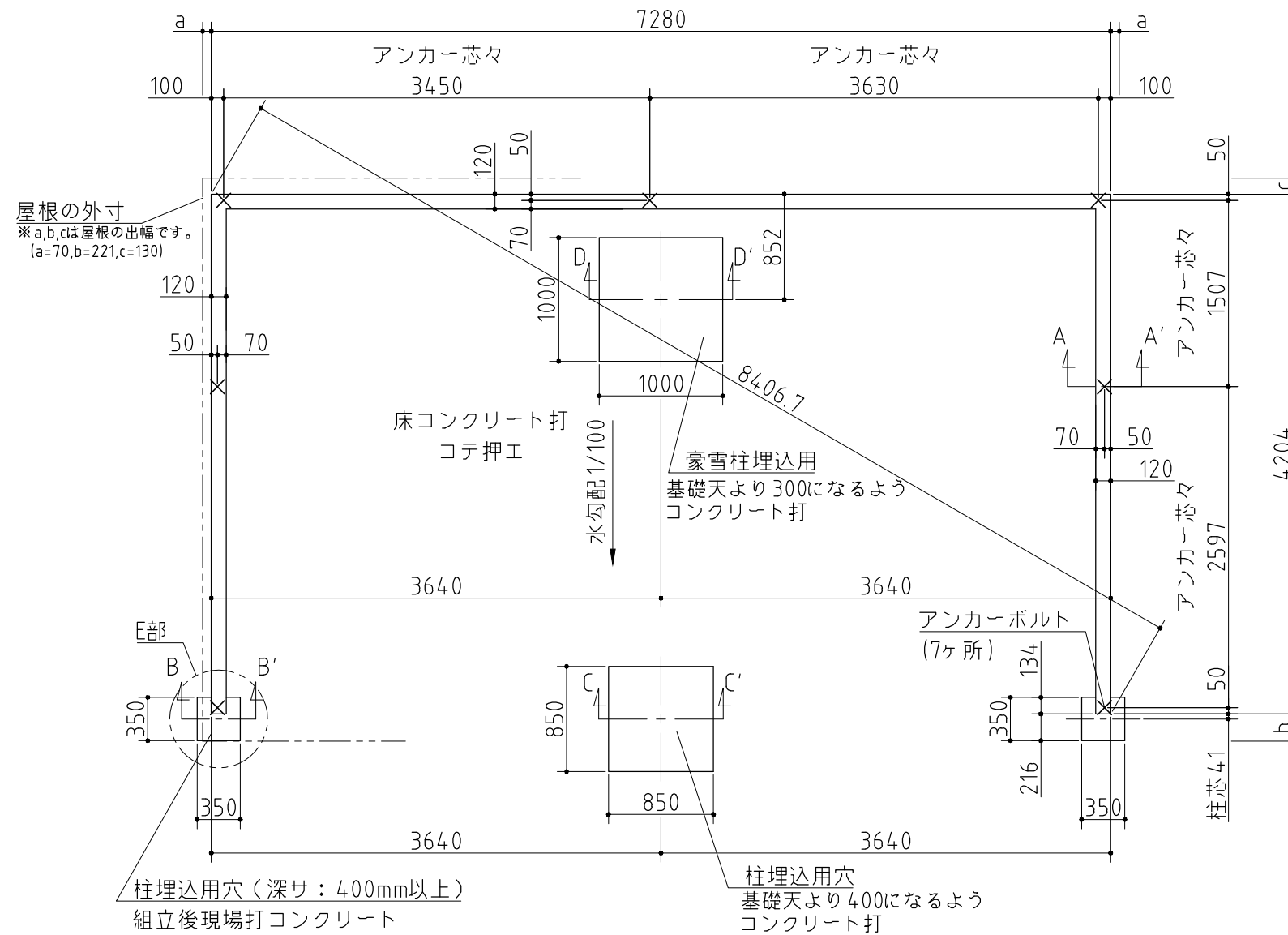
基礎詳細図 S=1/20
